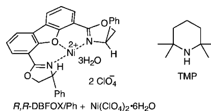
R,R -DBFOX/Ph + Ni(ClO 4 ) 2 ·6H 2 O
